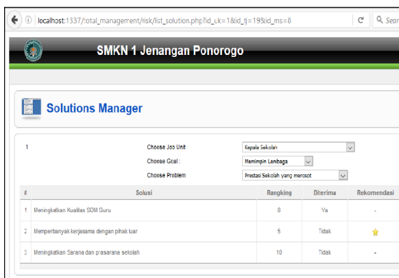
Gambar 14 Form entry solusi dan solusi yang diambil dari tiap masalah
