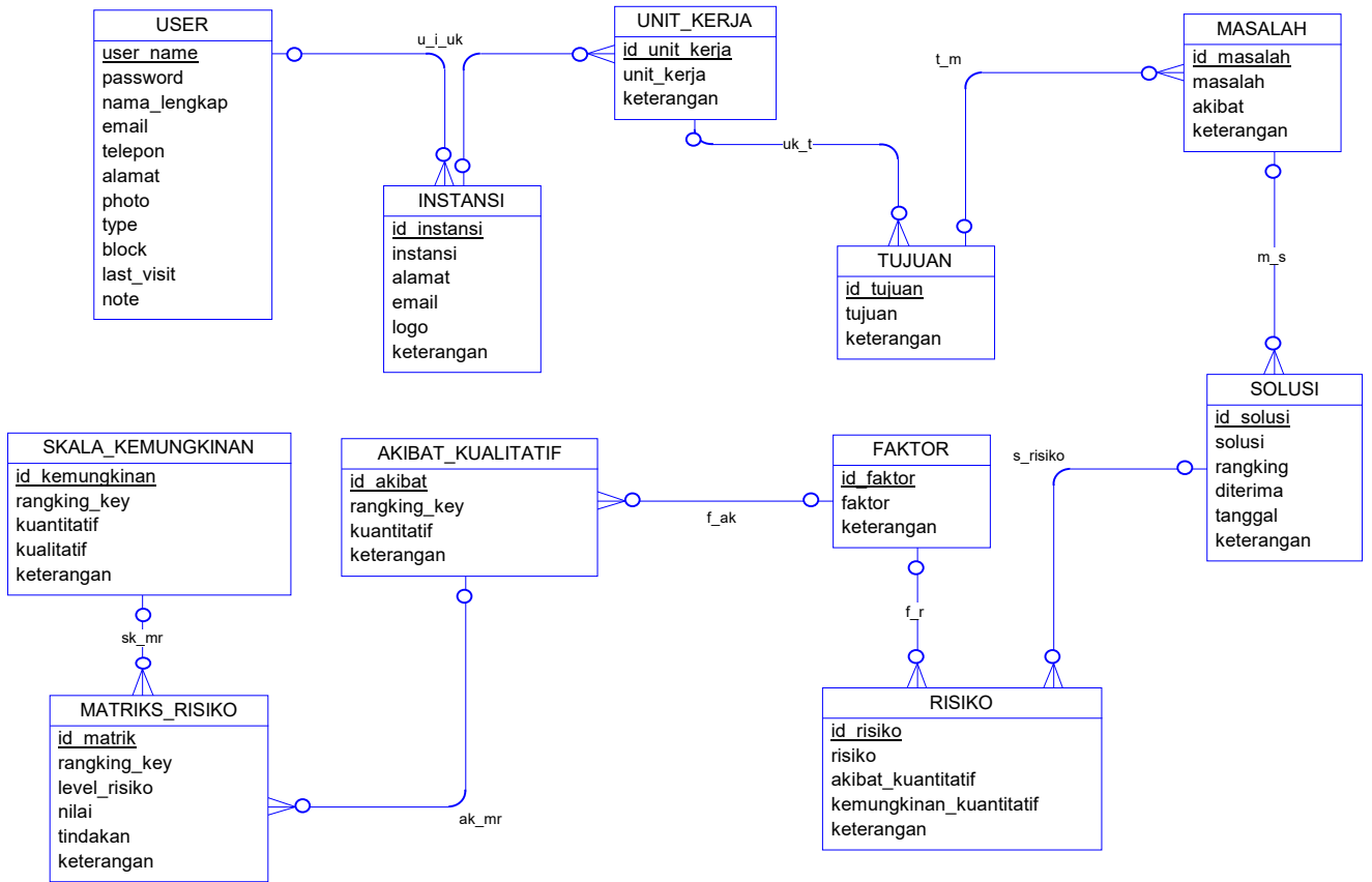
Gambar 6 Conceptual Data Manager Aplikasi Analisis Manajemen Resiko
