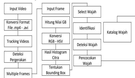
Gambar 1. Tahapan Deteksi Wajah
